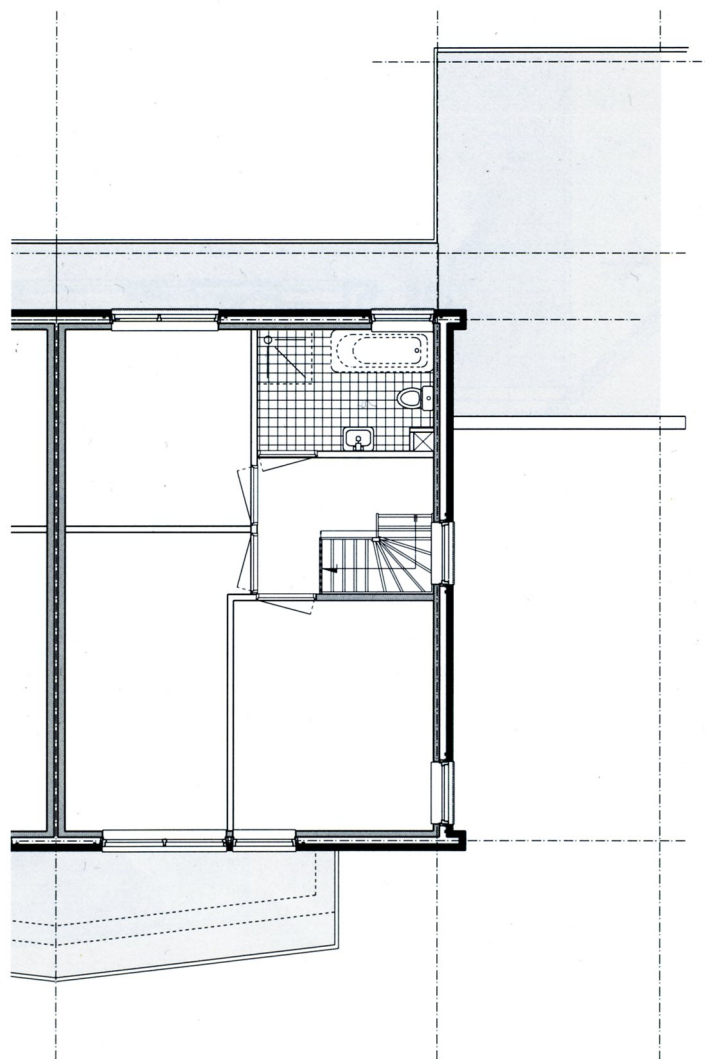
Verdieping
