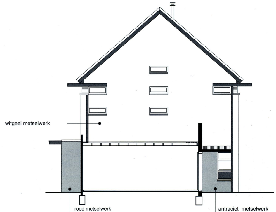
Kopgevel Z1
