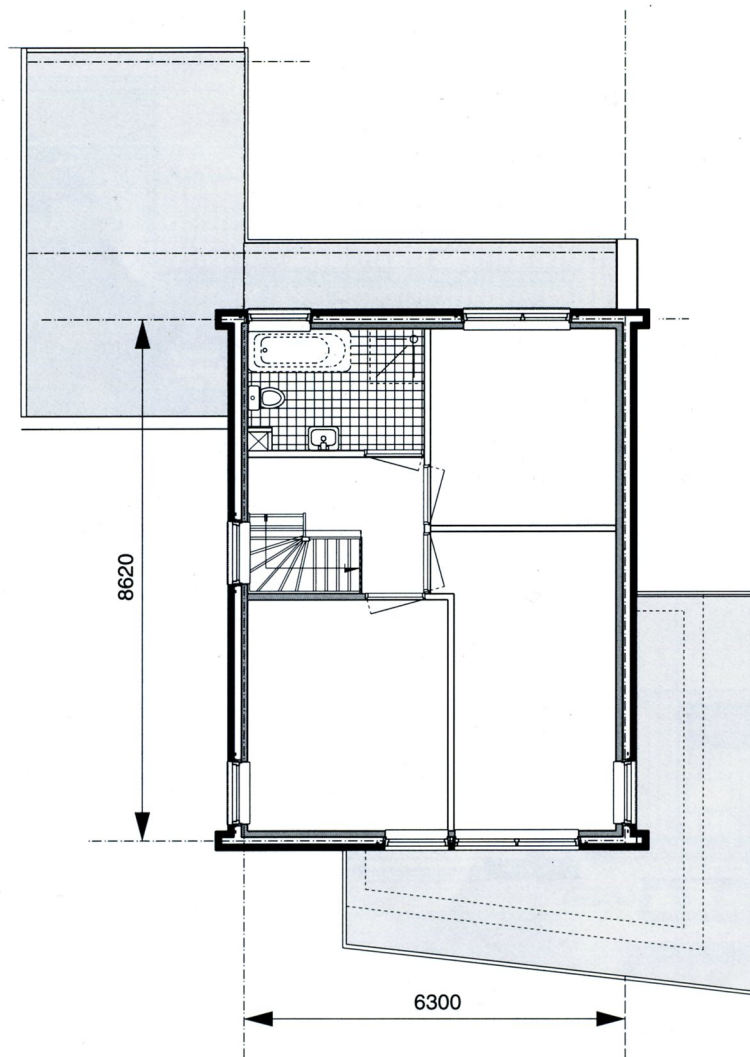
Verdieping type
