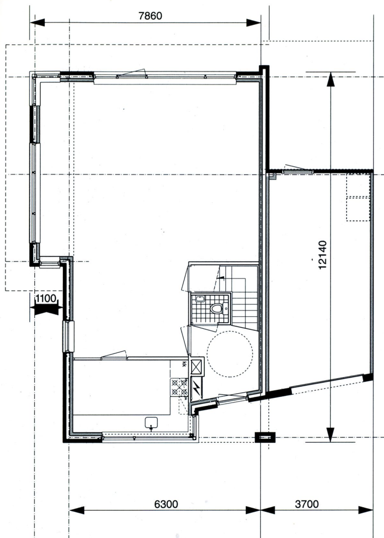
Begane grond
