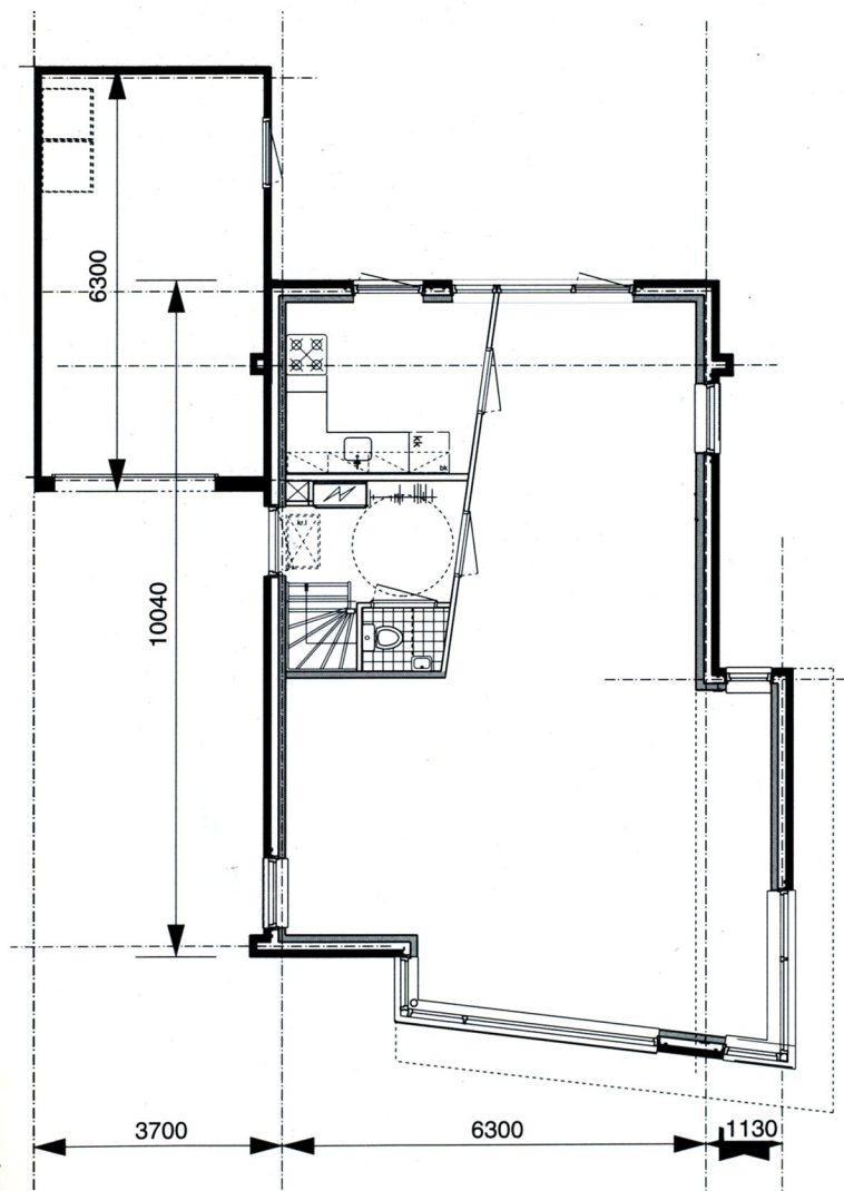
Begane grond
