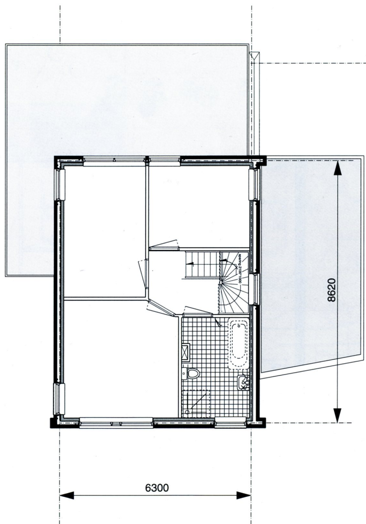
Eerste verdieping
