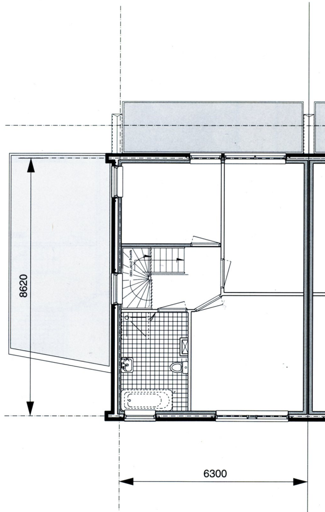
Eerste verdieping
