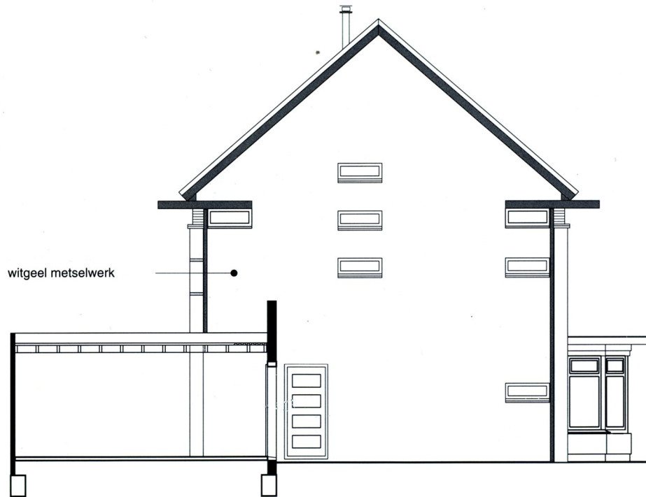
Kopgevel N1
