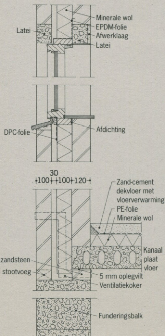
Gevelopbouw
