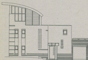
Noordgevel
