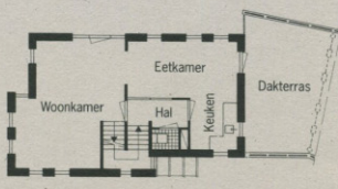
Verdieping
